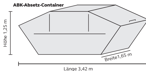
ABK-Absetz-Container
